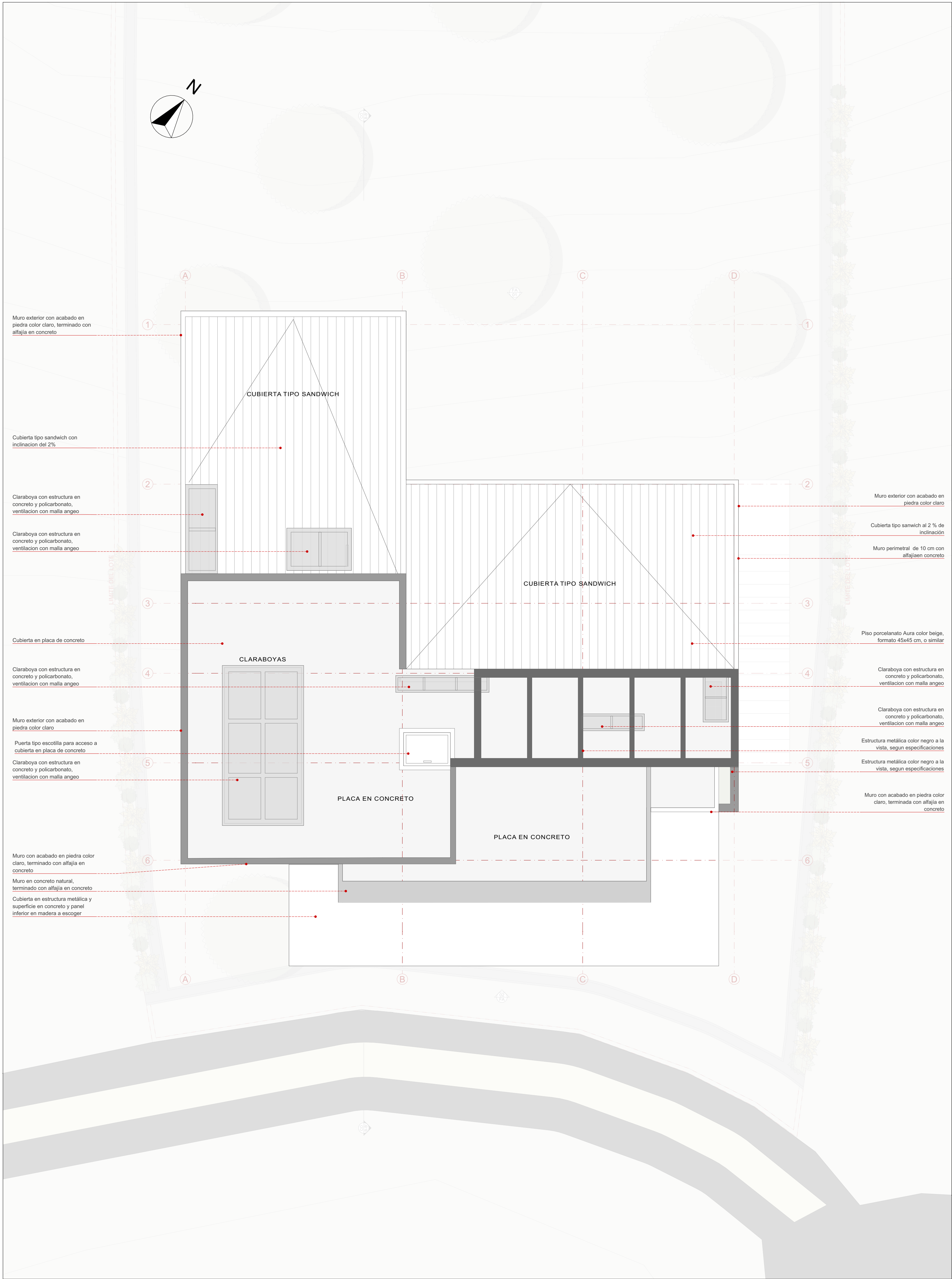
Plano de Cubiertas:
